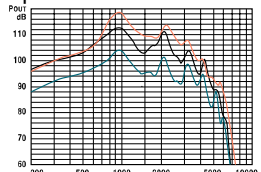
Entrada 31.6 mA/m CV: RTP
