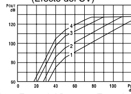
Unison Essential Potente: Entrada en 2000 Hz CV: como se muestra
