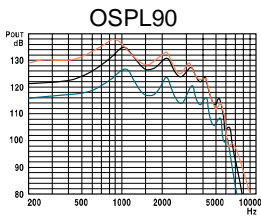
Nivel de Presión Sonora de Entrada: 90 dB CV: Máximo
