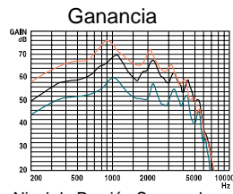
Nivel de Presión Sonora de Entrada: 50 dB CV: Máximo
